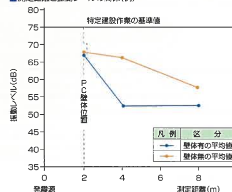
■ 測定距離と振動レベルの関係(例)
