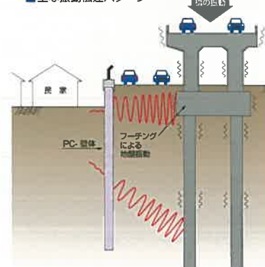
■ 主な振動伝達パターン
