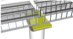
掛け違い部の橋脚
